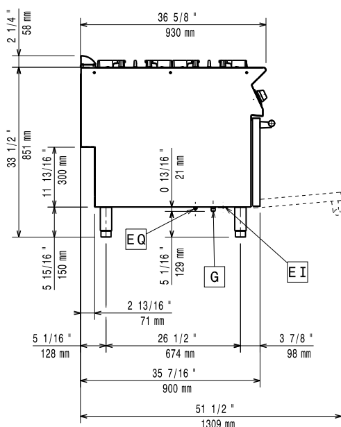
Oldalnézet
